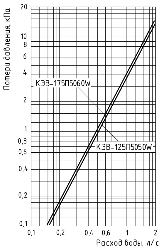
Рисунок 1. Гидравлические характеристики
